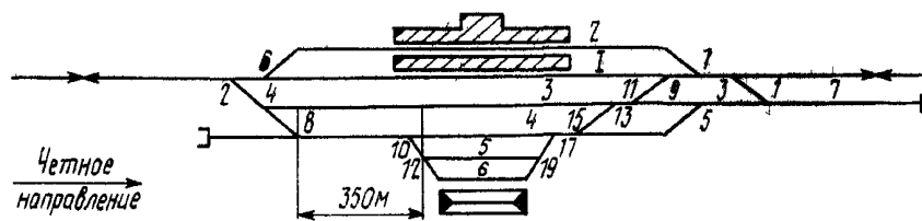
Рисунок 1 - Схема промежуточной станции
